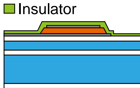
図 1.6 PE-CVD による酸化膜成膜
